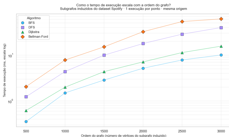
Figura 5 — Dispersão Ordem do Grafo \times Tempo de Execução (escala log). A distância entre a linha do Bellman-Ford e as demais cresce com a ordem do grafo.
