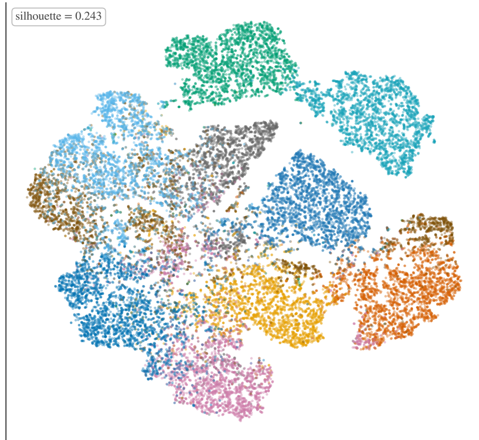
t-SNE
