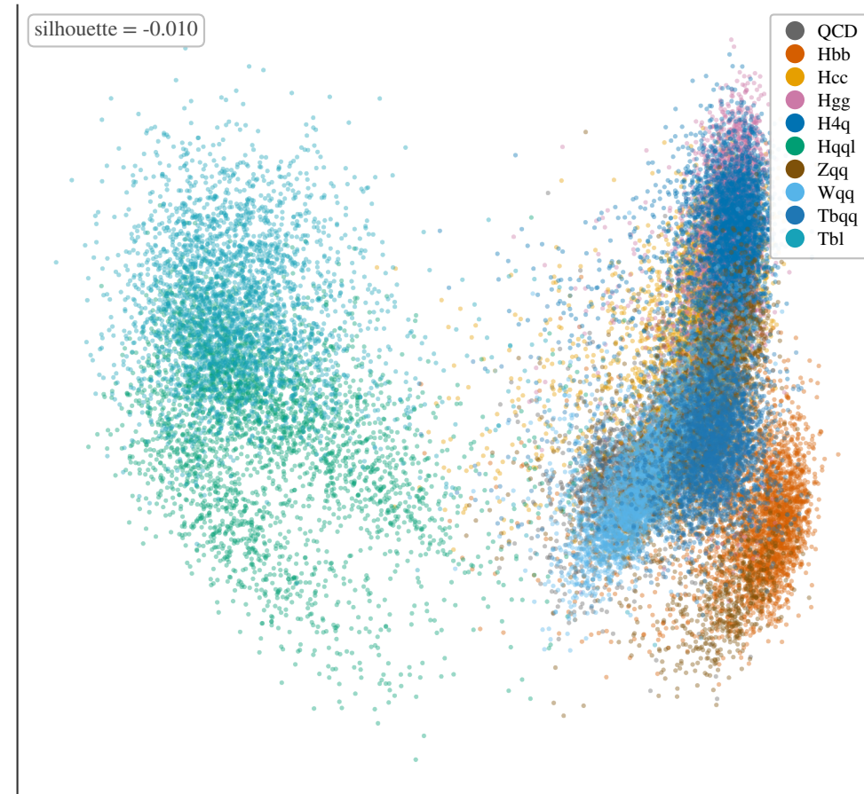
PCA
