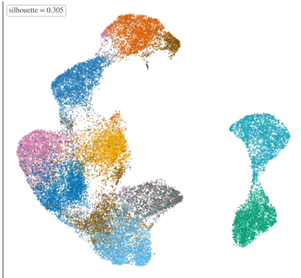
UMAP
