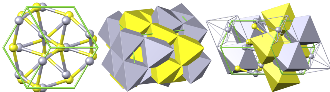
Figura 1: La struttura cristallina del cinabro
