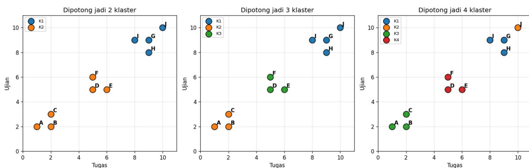
Gambar 4.8 Perbandingan Pemotongan Dendrogram menjadi 2, 3, dan 4 Klaster
