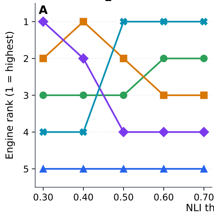
PAWC_norm rank
