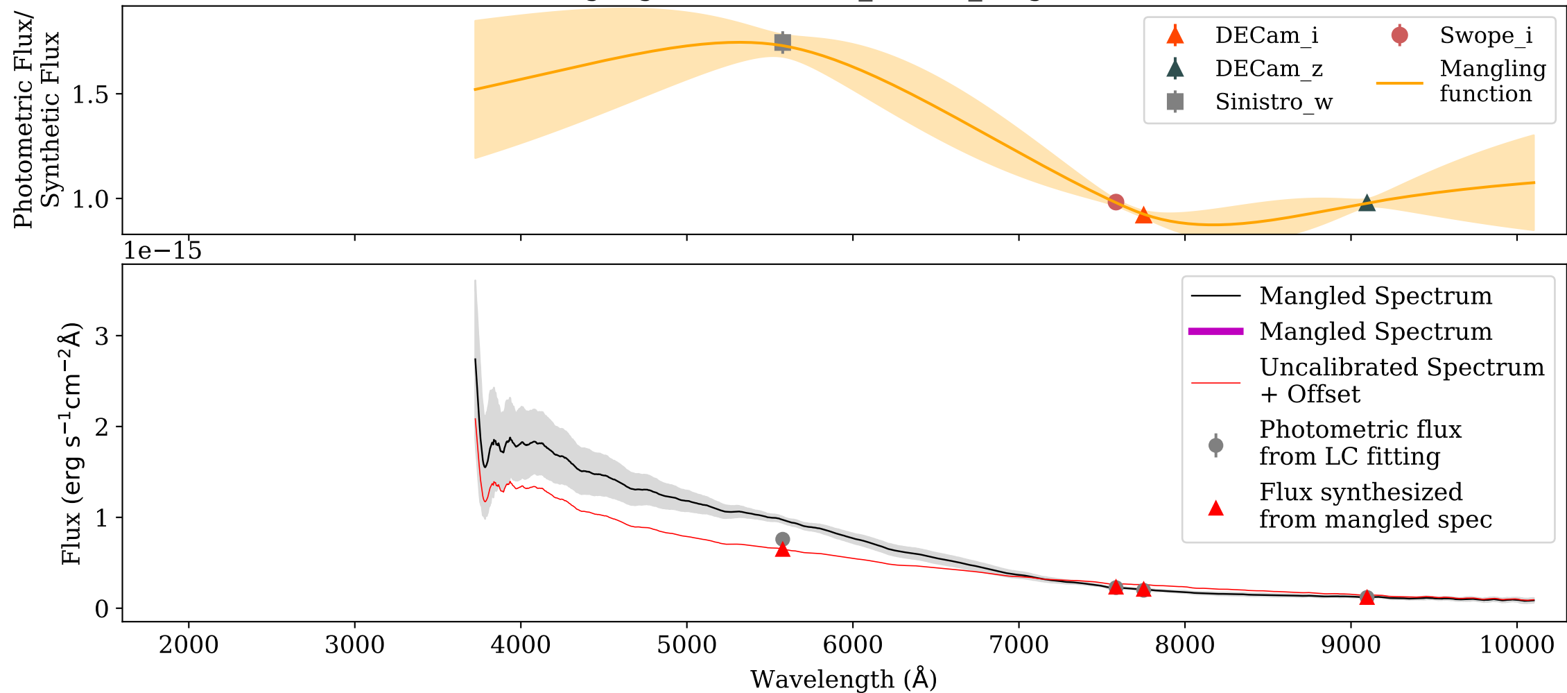
Mangling: 57983.01825_LDSS3_Magellan.dat
