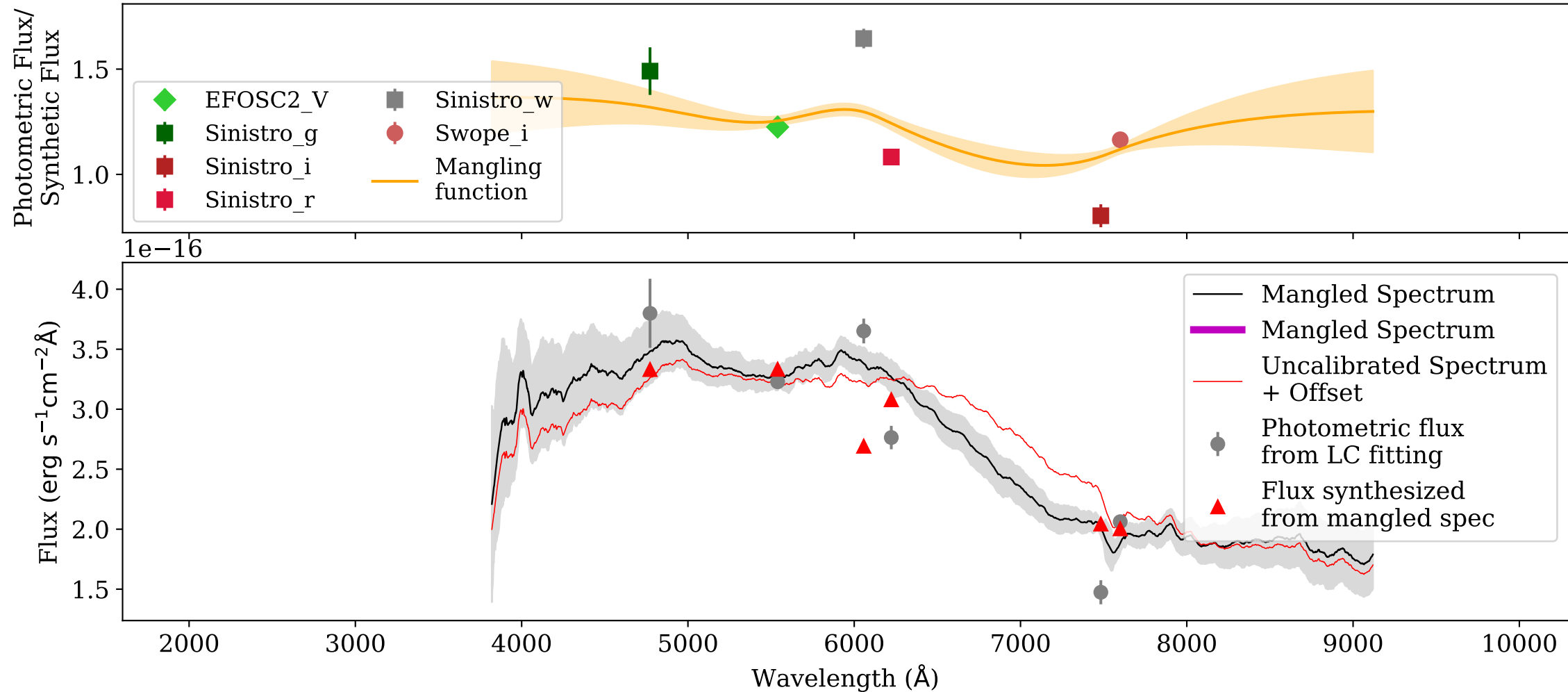
Mangling: 57983.9914_LDSS3_Magellan.dat
