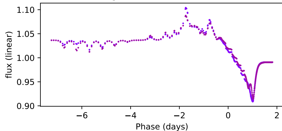
\log_{10}(wl) : 0.735-1.575
