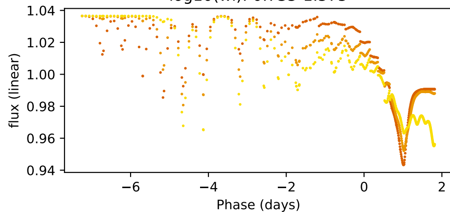
\log_{10}(wl) : 0.735-1.575
