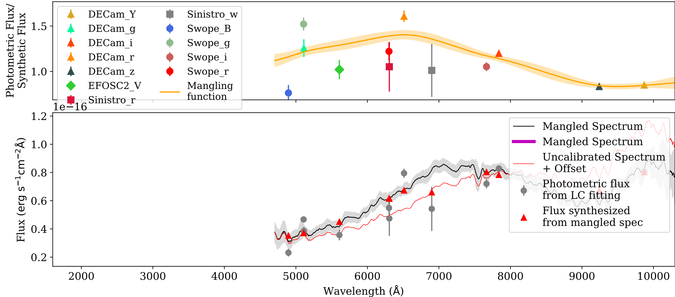
Mangling: 57985.99019_LDSS3_Magellan.dat
