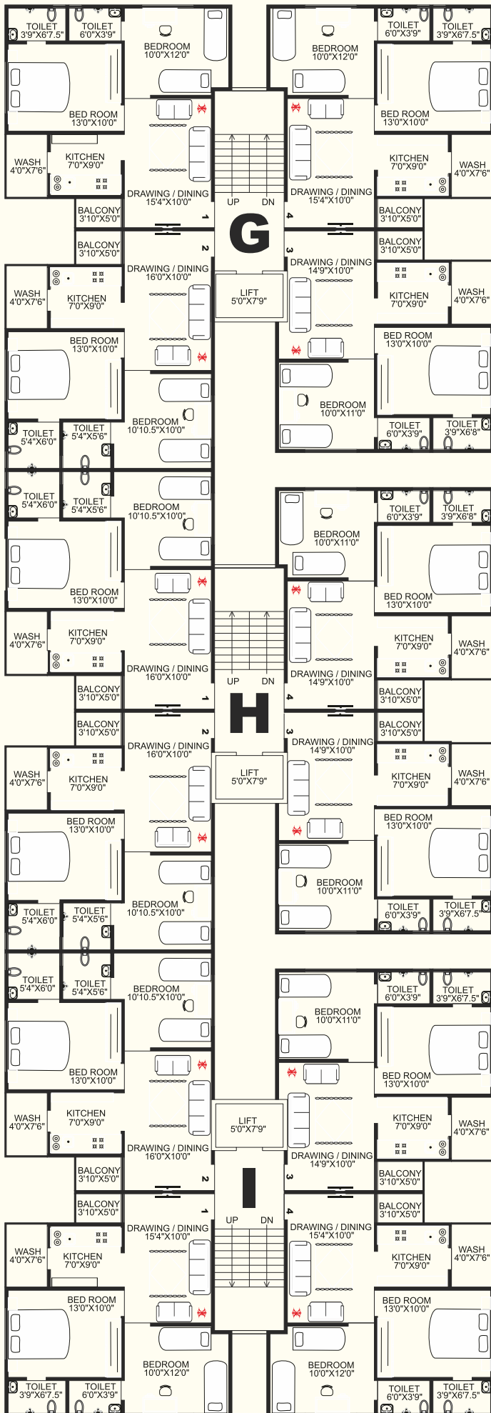
Typical Floor Plan (G.F.,F.F.,S.F.,T.F.)
