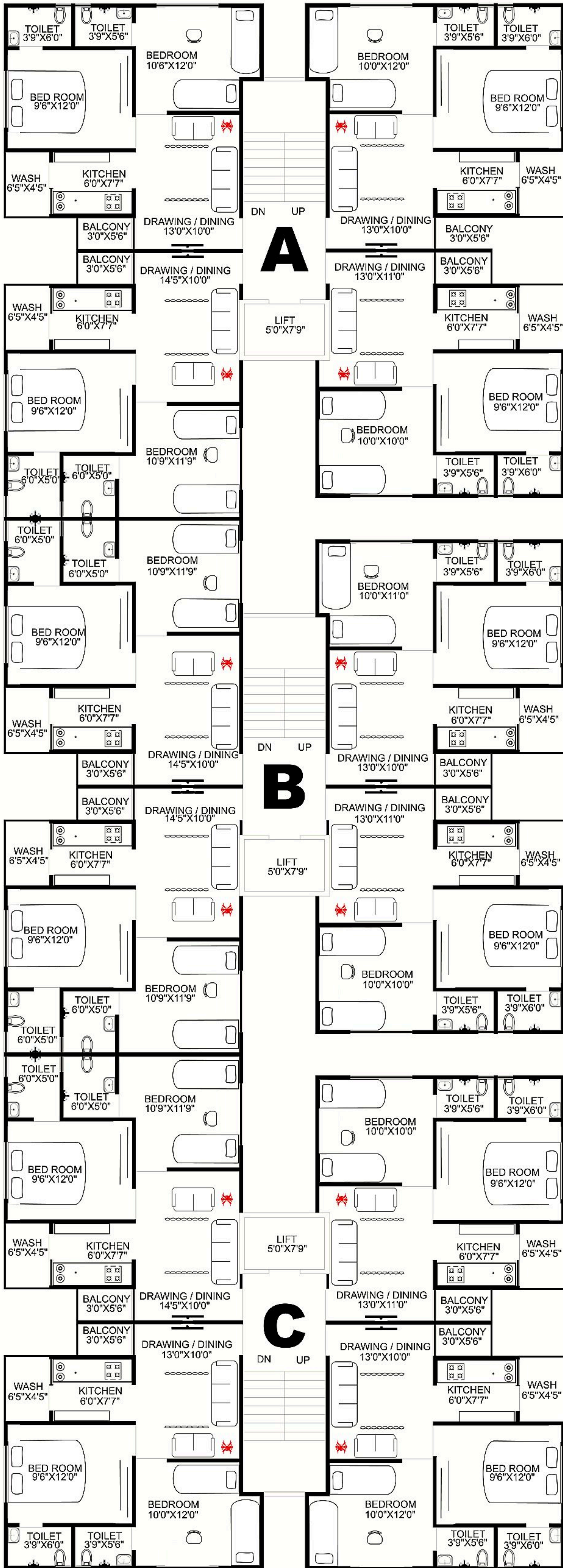
Typical Floor Plan (G.F., F.F., S.F., T.F.)
