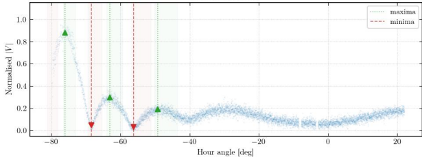
ch 655 (10.450 GHz)
