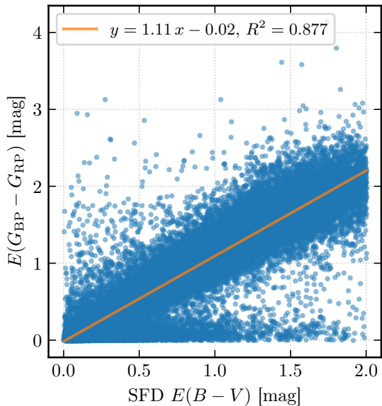
SFD \leq 2.0 mag
