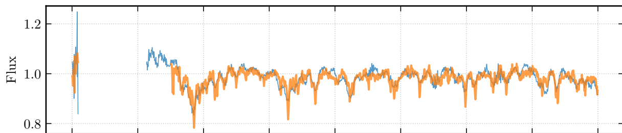
2M19431273+2445286
