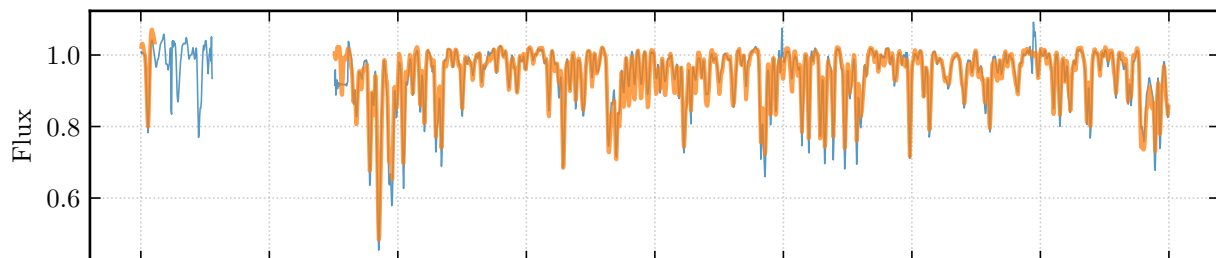
2M19465744+2511396
