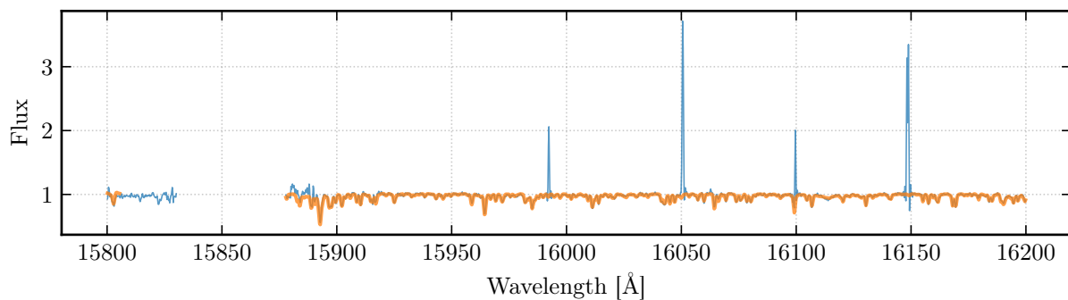
2M21344249+1214085
