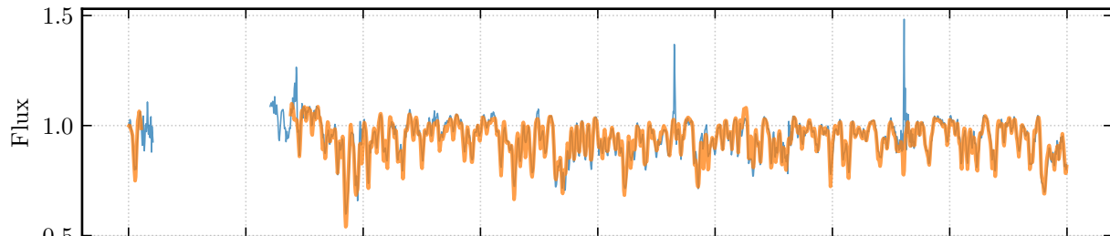
2M21281377+1054307
