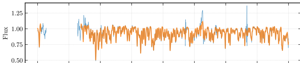
2M21344249+1214085
