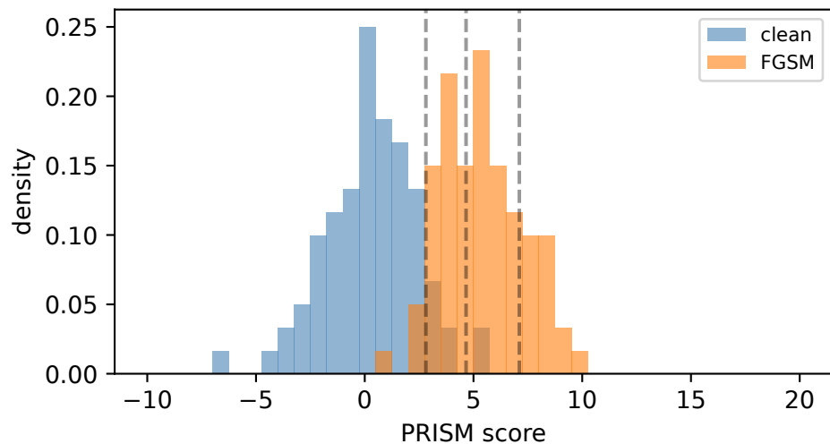
FGSM (TPR L1=0.93)
