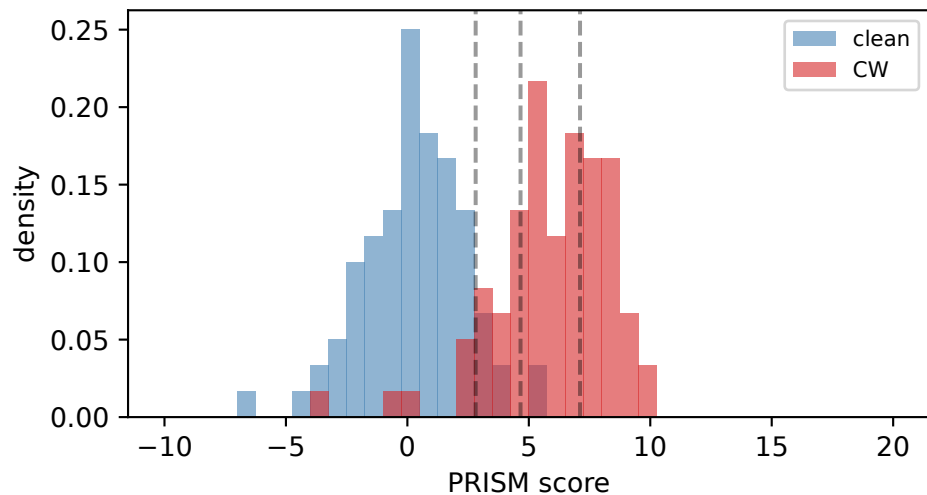
CW (TPR L1=0.93)
