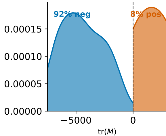
GPT-2 355M
