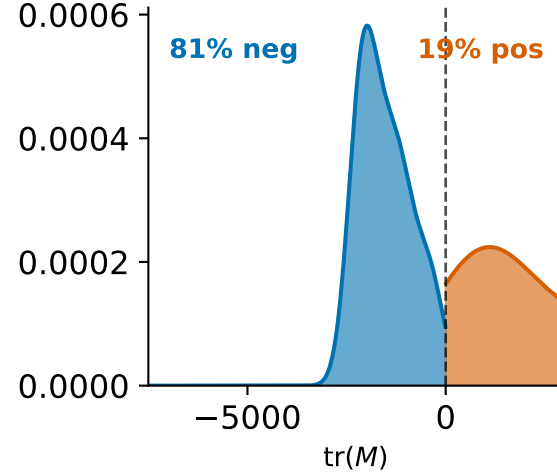
GPT-2 774M
