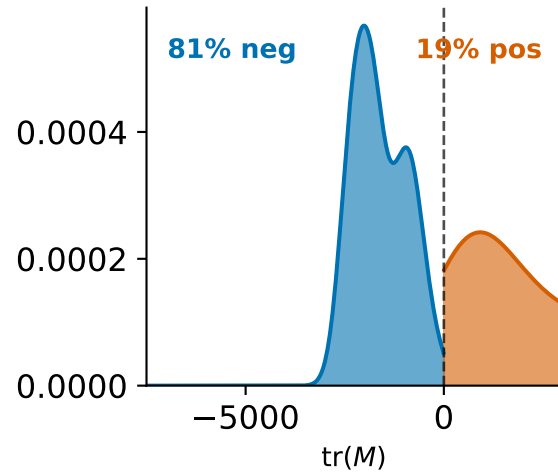
GPT-2 1.5B
