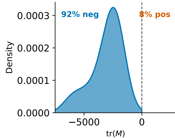
GPT-2 124M
