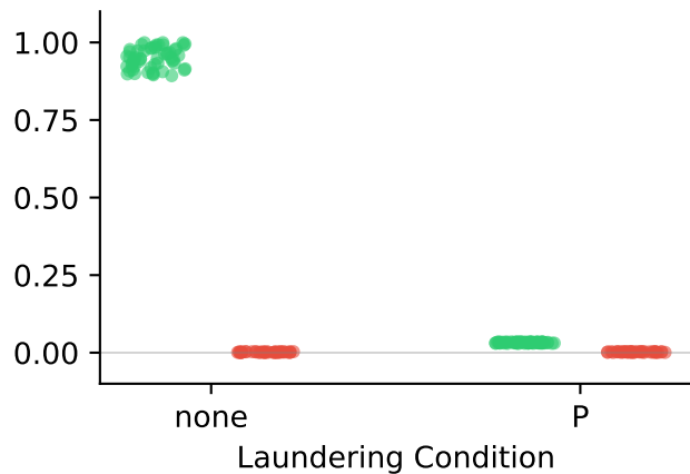
(d) GPT-2: Weight Cosine
