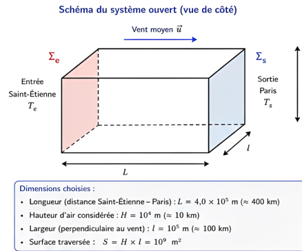
Figure 1: Système ouvert en convection
