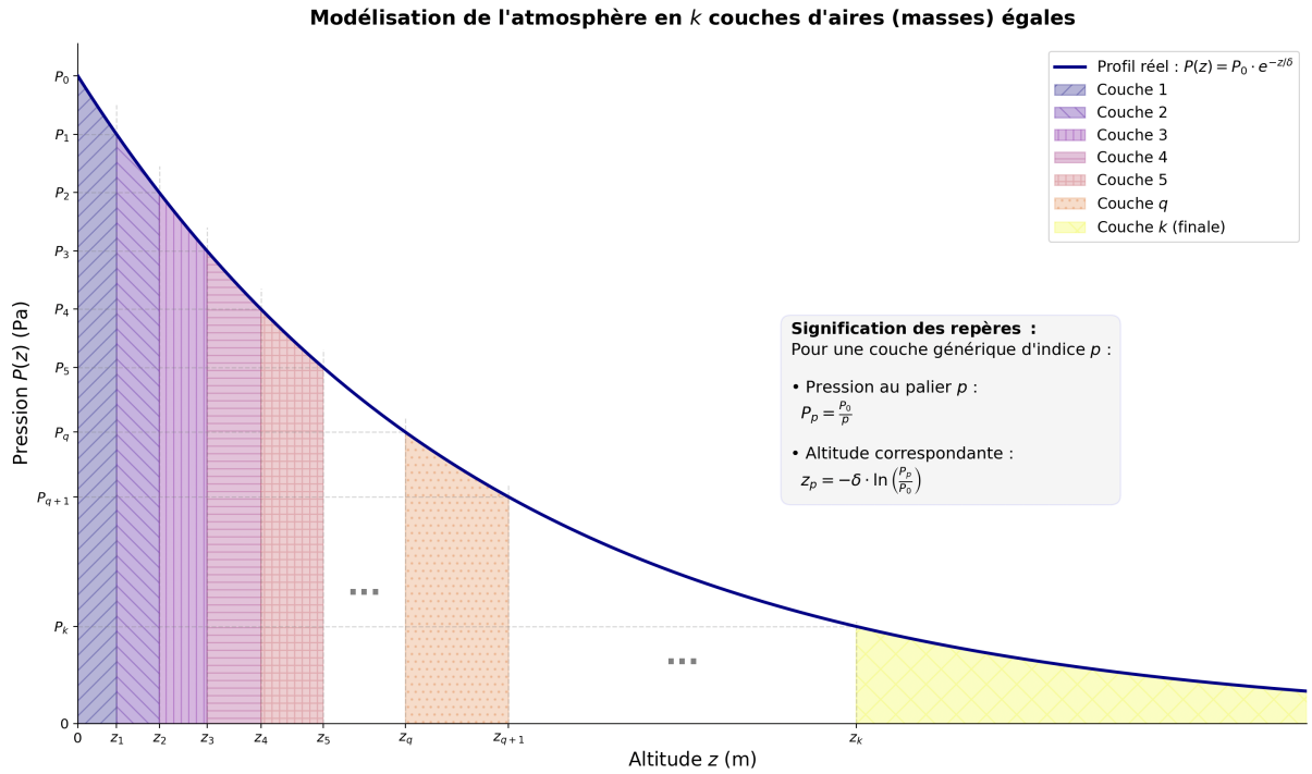
FIGURE 4 – Profil exponentiel de pression et découpage en k couches de masse identique.
