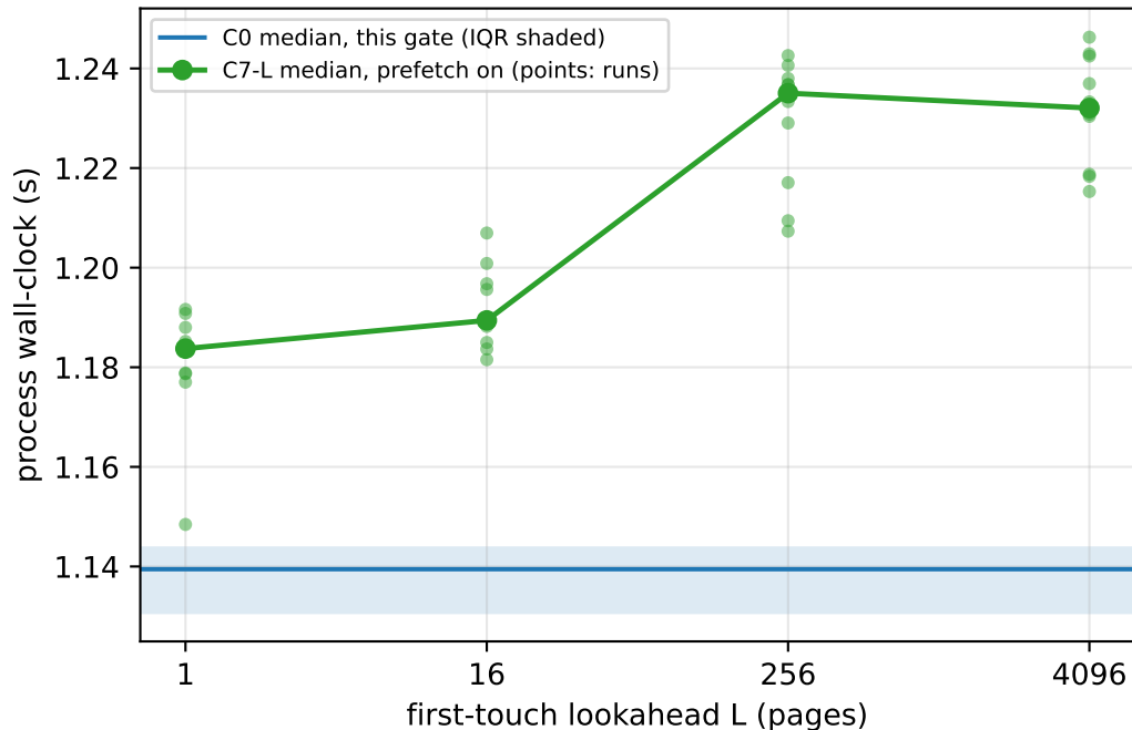
Stencil-24K (n=10 per cell)
