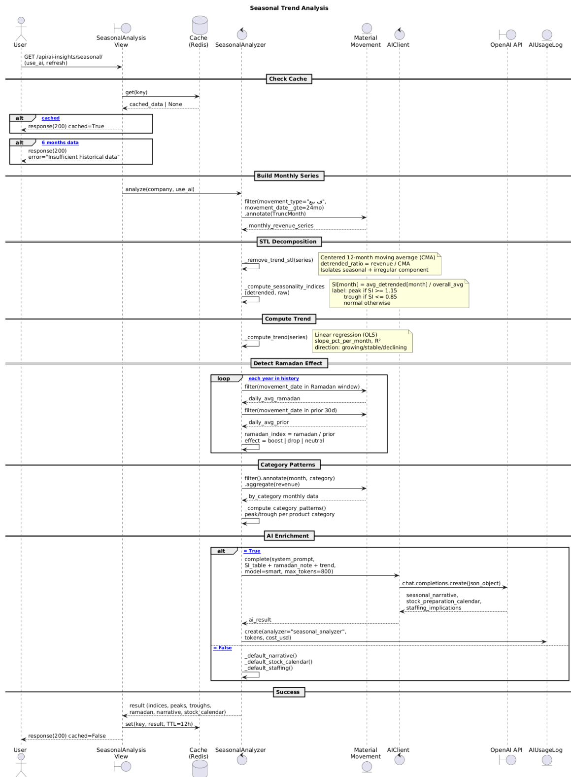
FIG. 6.3: Diagramme de séquence de conception — Analyse des tendances saisonnières
