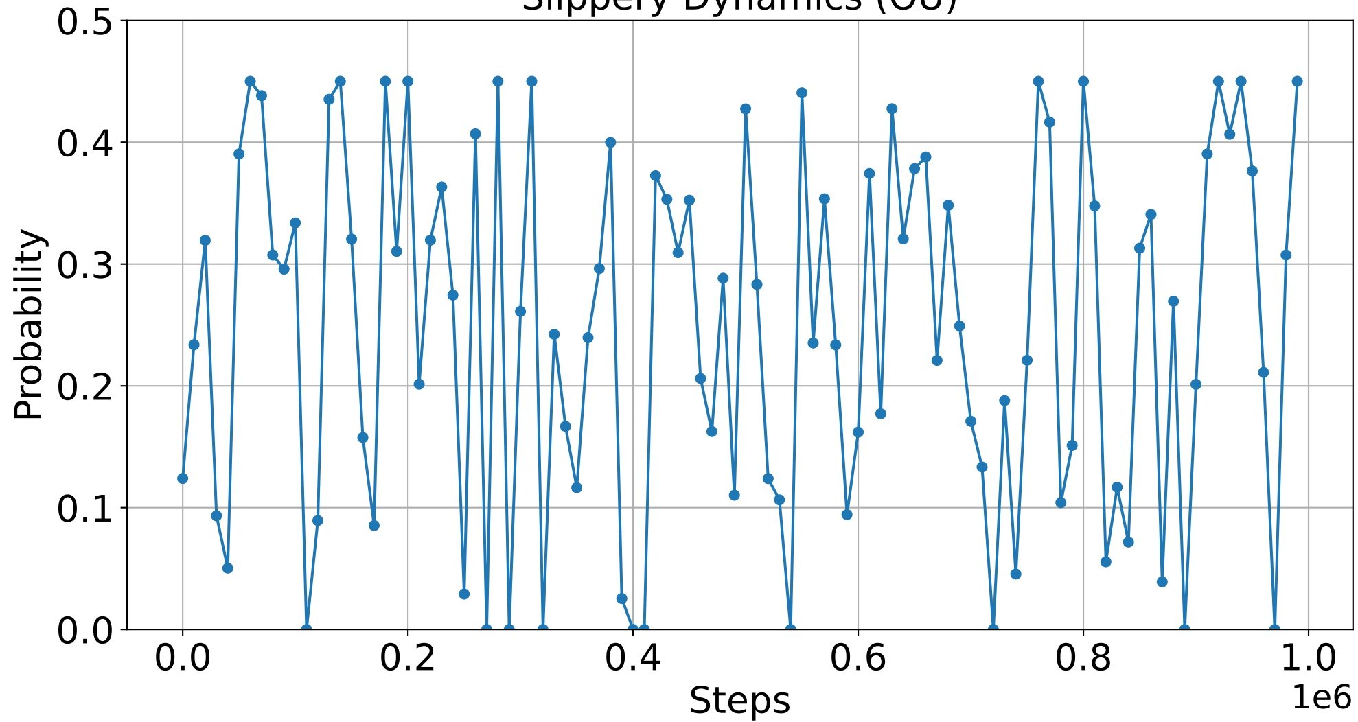
Slippery Dynamics (OU)
