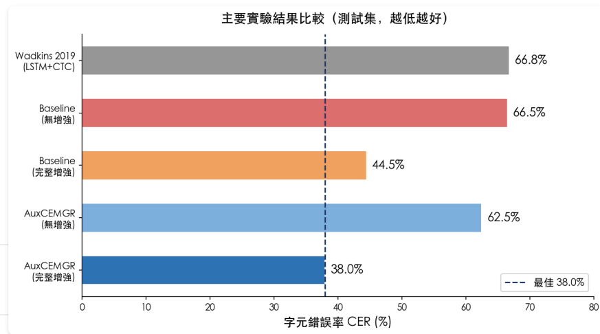
主要結果橫條圖 (越低越好)
