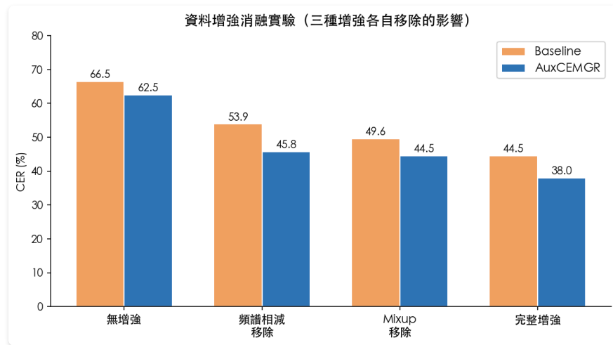
三種增強各自移除後的 CER 變化
