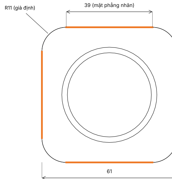
NHÌN TRÊN
