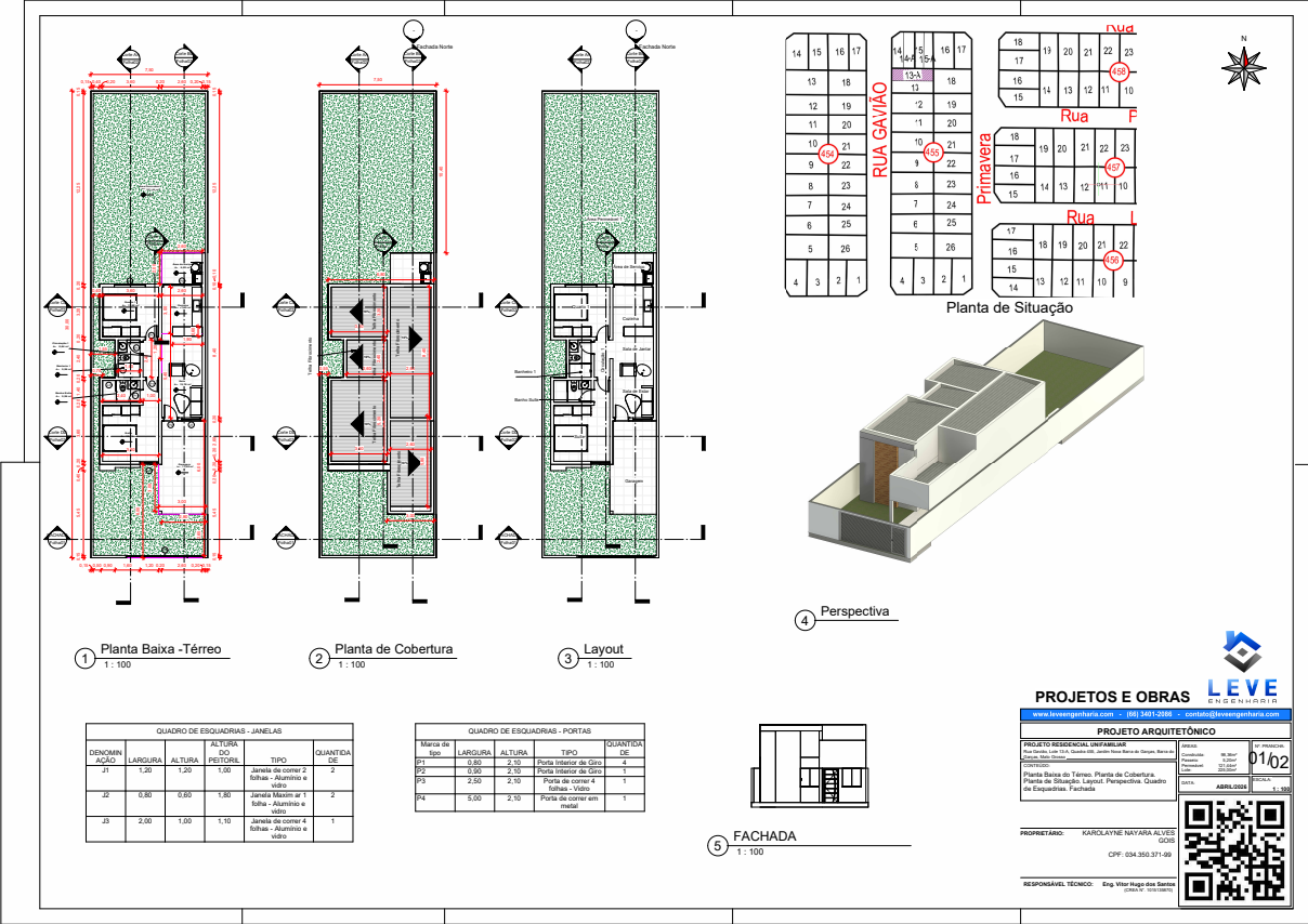
FIGURA 4 – Projeto arquitetônico (Planta Baixa; Perspectivas).
