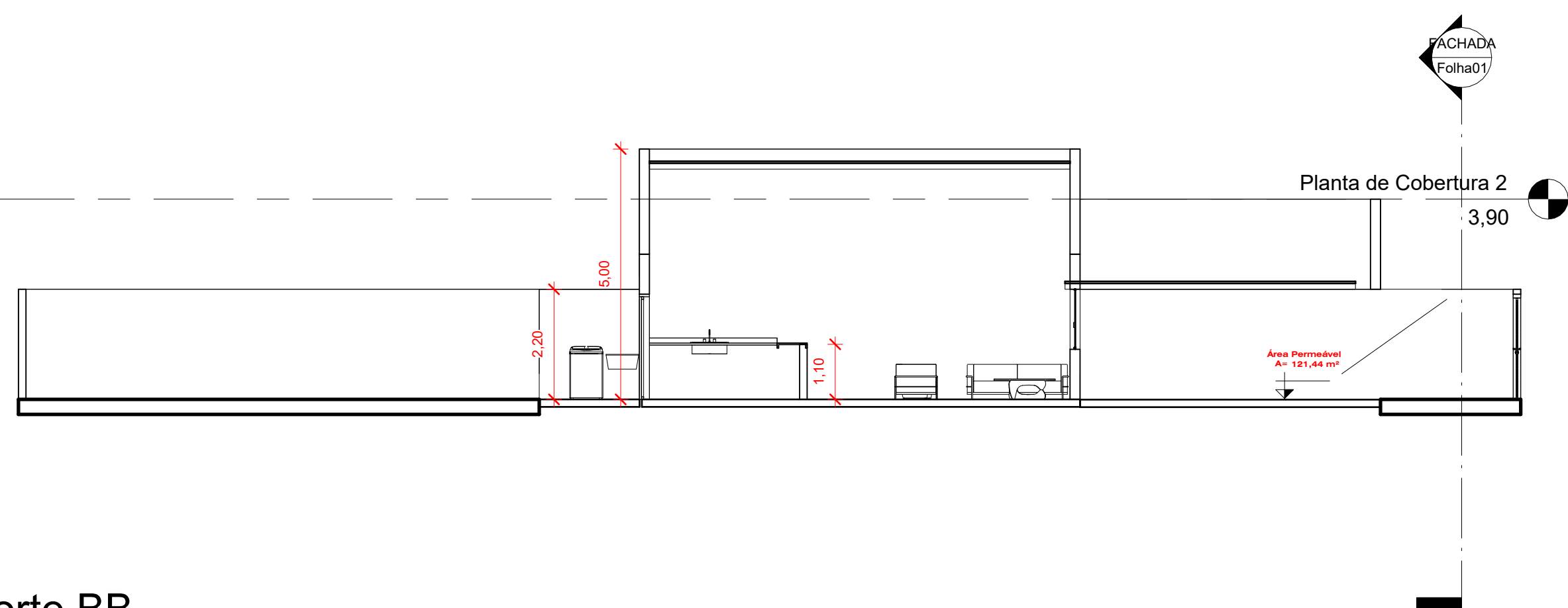
2 Corte BB 1 : 100
