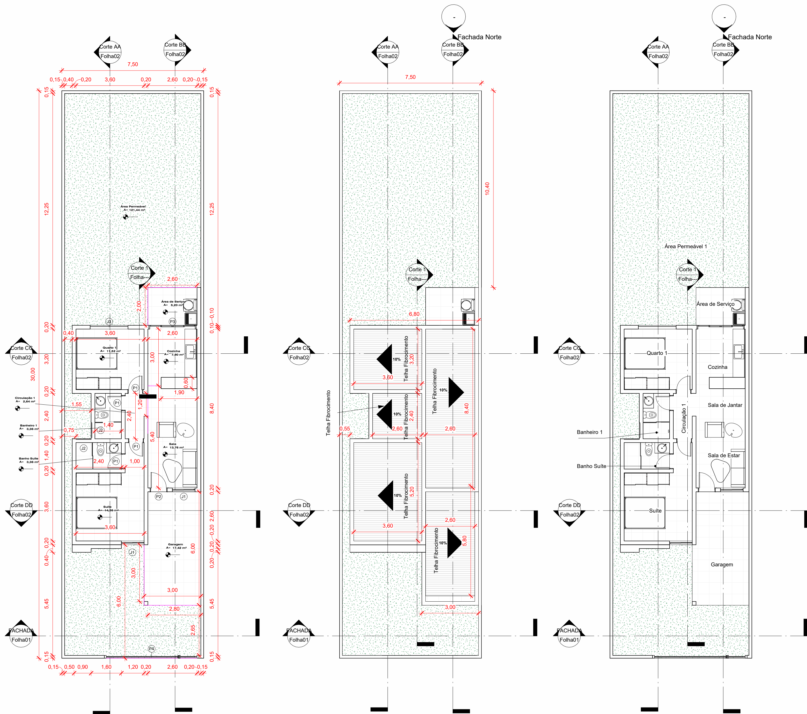
1 Planta Baixa -Térreo 1 : 100
