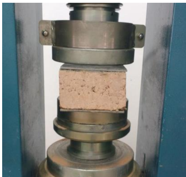
FIGURA 6 – Corpo de prova no ensaio de resistência à compressão
