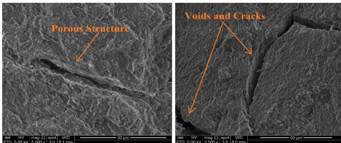
Figura 1 – Solo tratado com cimento após 28 dias de cura.
