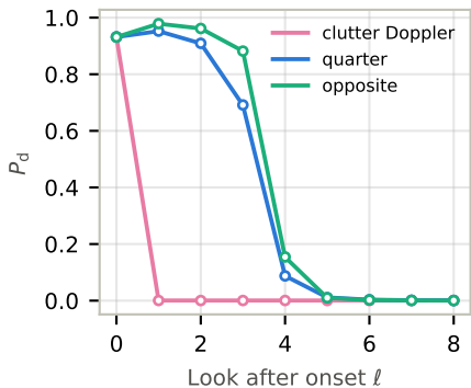
(d) Whitenized non-coherent integration
