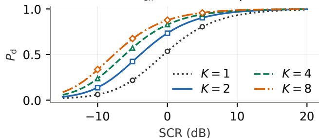
(d) Whiten noncoherent integration Power: K_{\text{eff}} = 1.41 over 8 pulses
