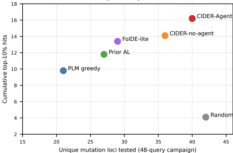
Quality-diversity frontier
