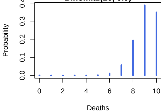
Binomial(10, 0.9)
