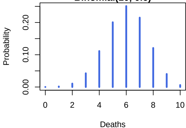
Binomial(10, 0.6)
