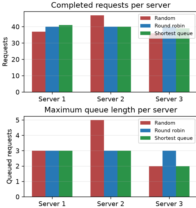
Figura 3. Distribuição final de requisições concluídas e maior fila observada por servidor na rajada representativa de 120 requisições.
