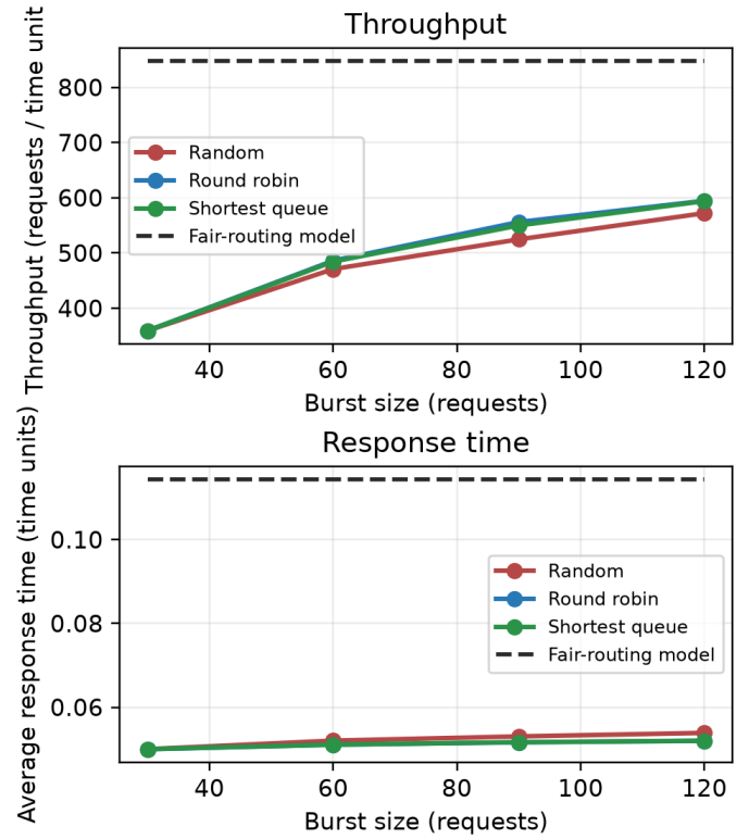
Figura 1. Vazão e tempo médio de resposta simulados, comparados ao modelo de roteamento justo.
