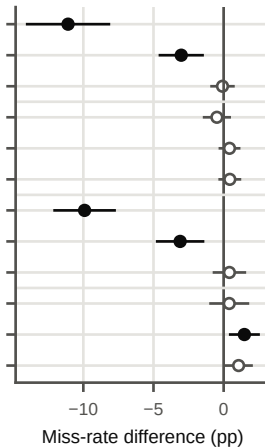
c H3: Diffusion-RB minus Diffusion-JCSO
