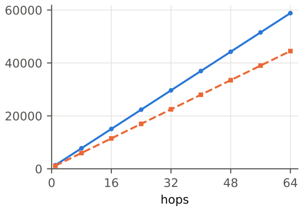
Transcript \text{hist}_n
