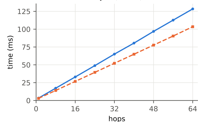
Identify (auditor)
