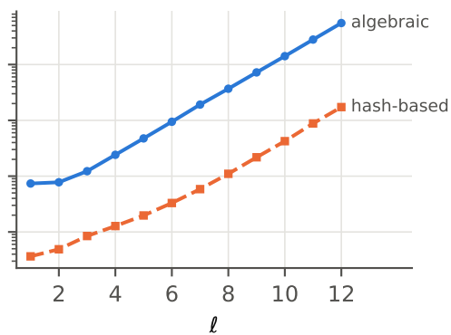
Trace (auditor)
