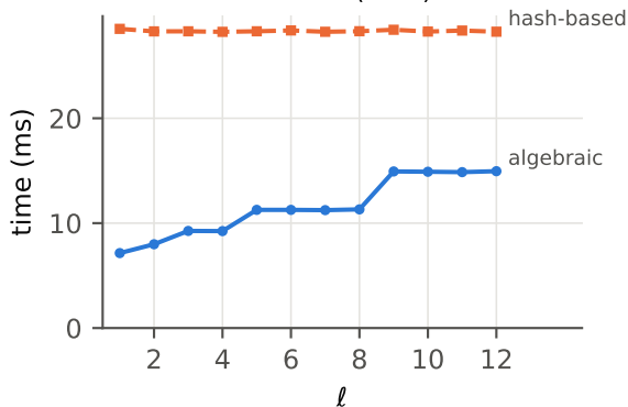
Submit (user)
