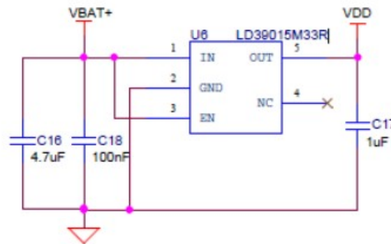
LDO
