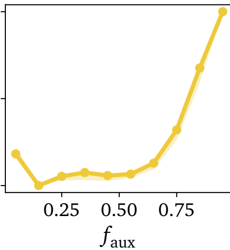
z_{aux} (latent 195)
