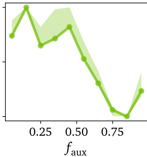
z_{bs} (latent 973)
