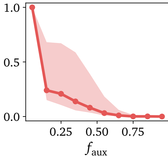
z_{bc} (latent 640)
