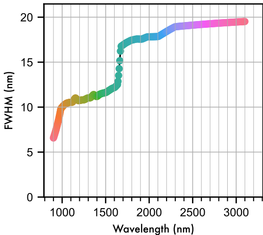
Enfys_Inas_Mwir_Snr10X FWHM
