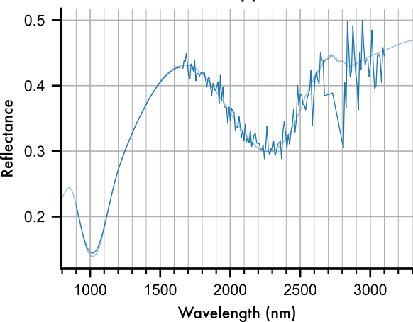
H. Nbpp22
