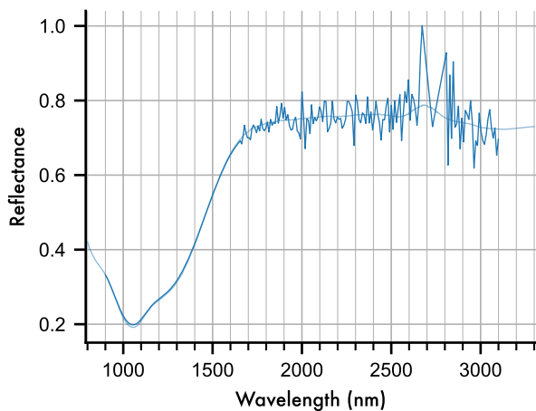
K. Lasc02
