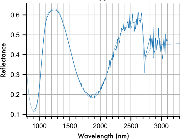
I. Lapp47B
