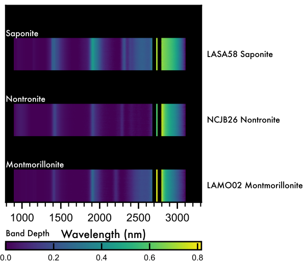
O. Smectites
