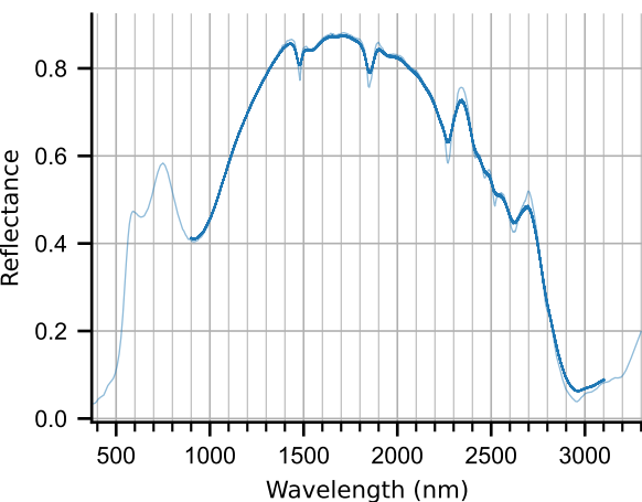
Jarosite
