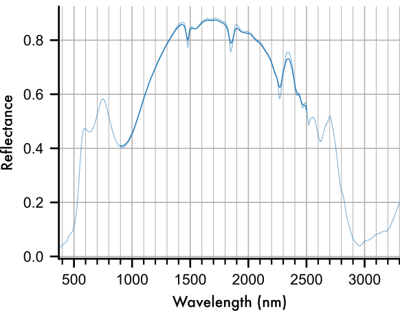
Jarosite
