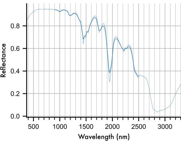
Gypsum
