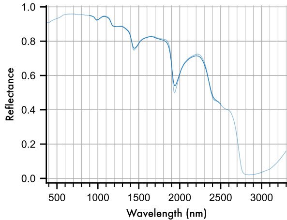
Mg-Sulphate
