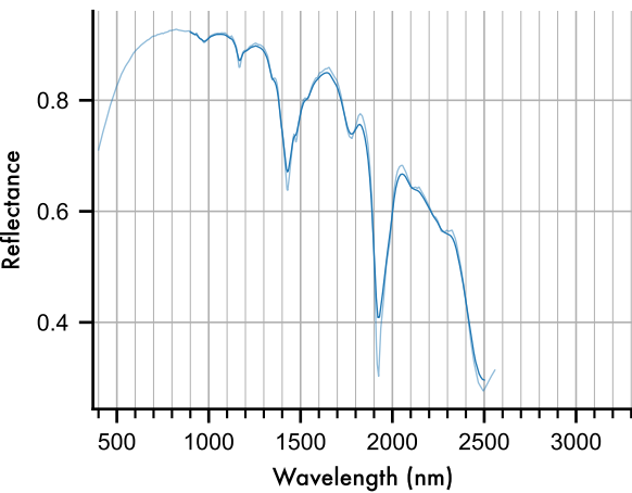
Bassanite
