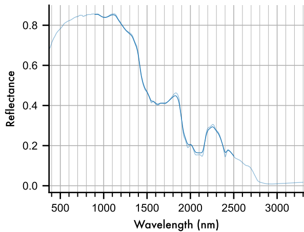
Kieserite
