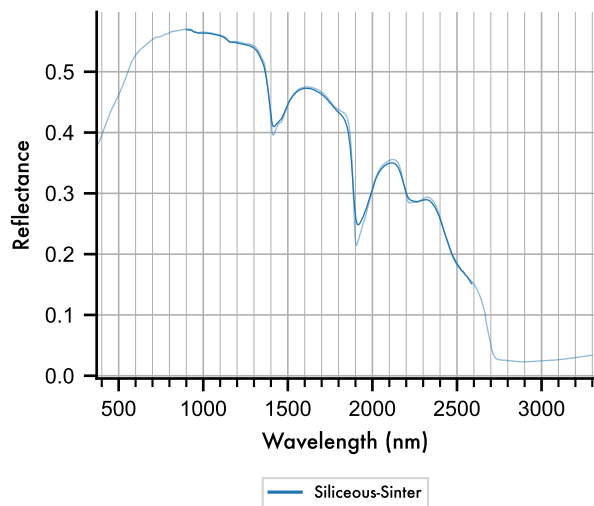
F. Gds26
