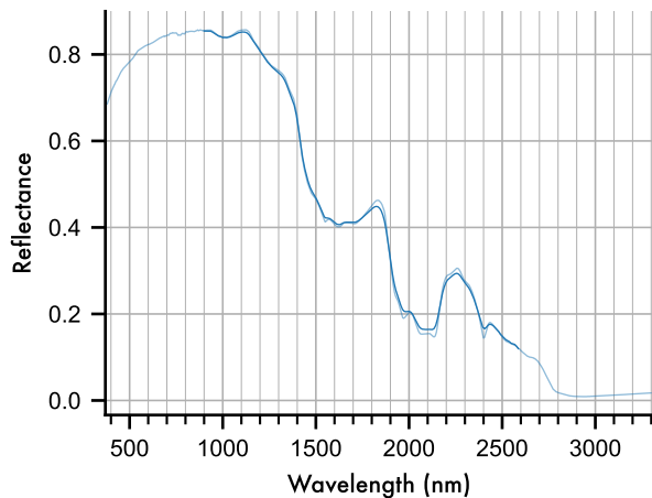
Kieserite
