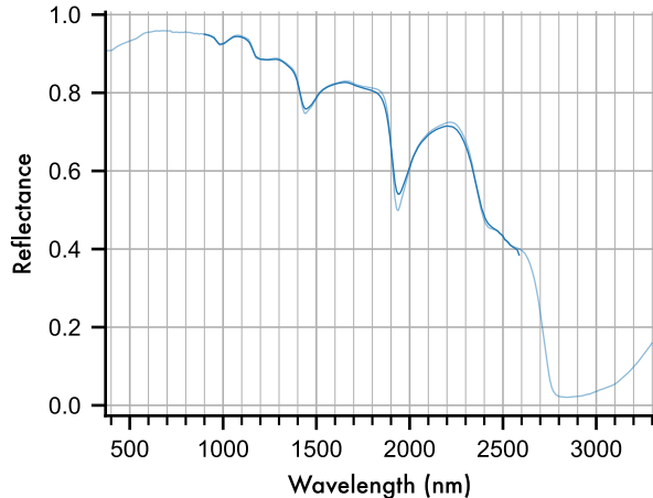
Mg-Sulphate
