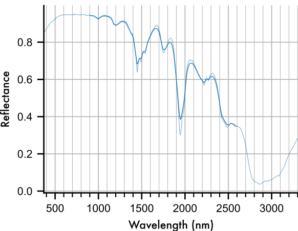
Gypsum
