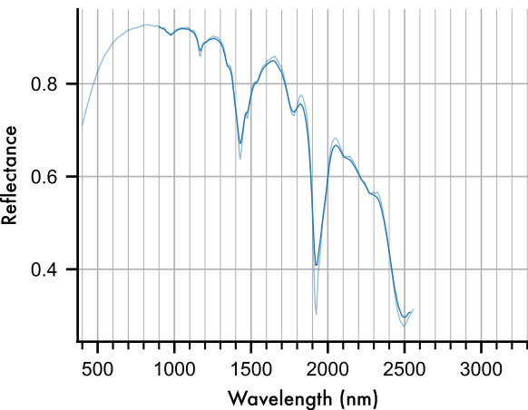
Bassanite
