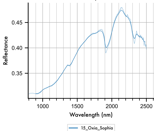
K. 15_Oxia_Sophia_00003
