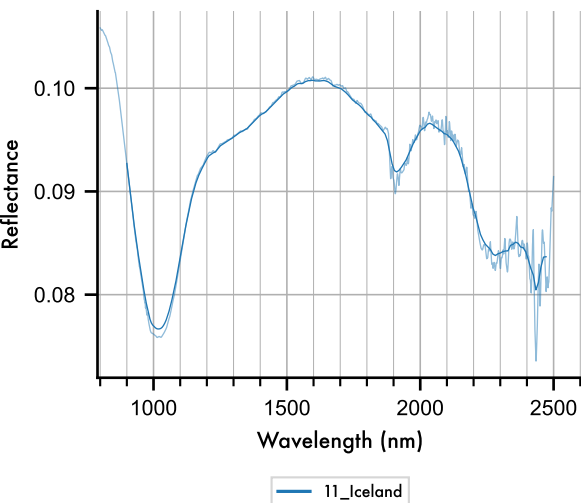
H. 11_Iceland_00004
