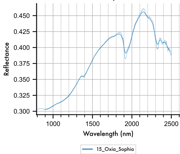
L. 15_Oxia_Sophia_00004
