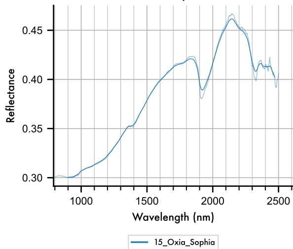
L. 15_Oxia_Sophia_00004
