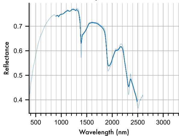
Vermiculite
