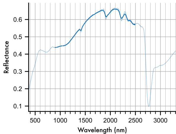
Illite
