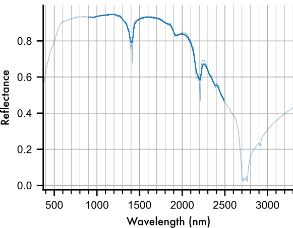
Kaolinite
