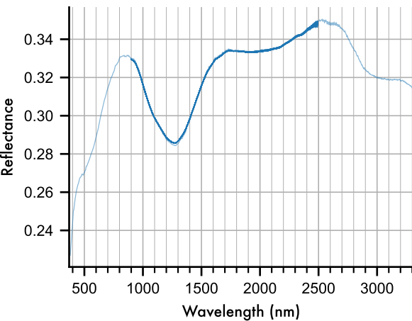
Plagioclase
