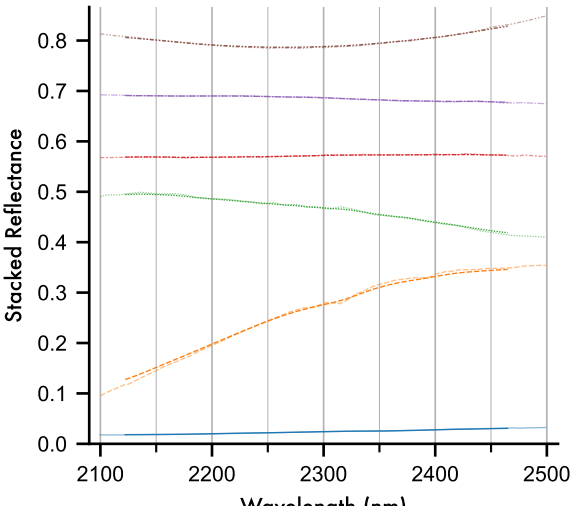
B. Sulfates
